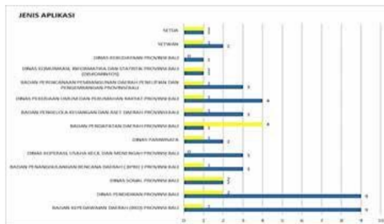
Gambar 6. Jenis Aplikasi
