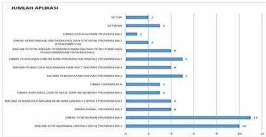
Gambar 2. Jumlah Aplikasi
